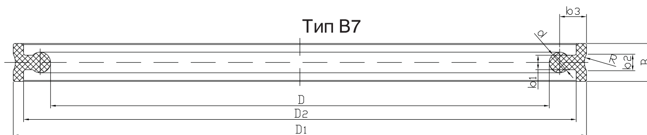
ОСНОВНИ РАЗМЕРИ (мм)
