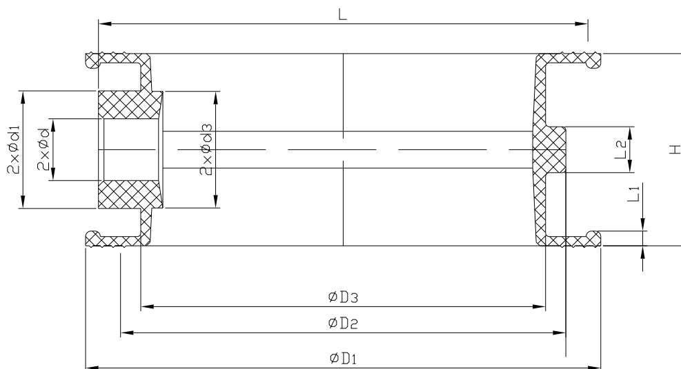
ОСНОВНИ РАЗМЕРИ (мм)
